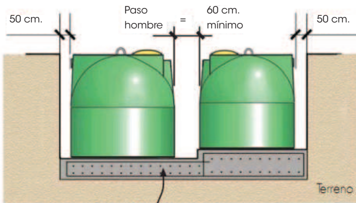
Ejemplo equipo depuración en polietileno
